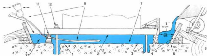
Рисунок 1: Схема применения MasterFlow 928 для высокоточной цементации оборудования
