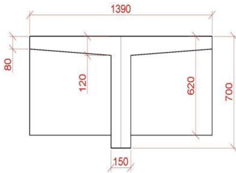
Рисунок Б.2 – Опалубочный чертеж балки
