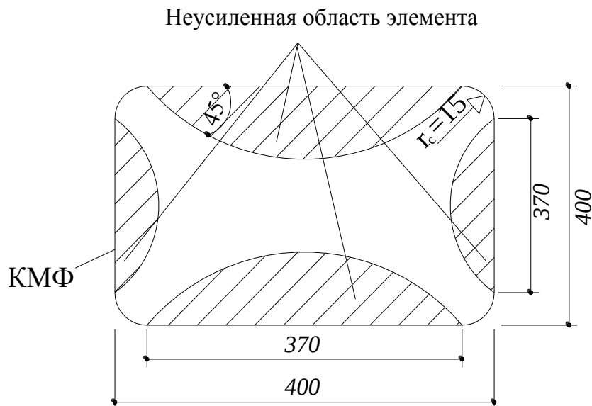
Рисунок В3 – Прямоугольная колонна обернутая по всей длине углеволокном
