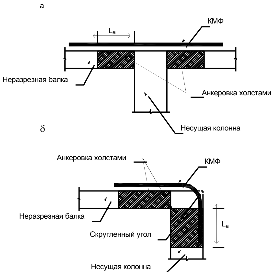
Рисунок 10 – Усиление и анкеровка неразрезных балок
