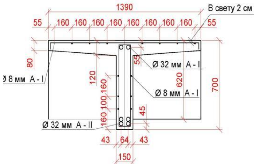
Рисунок Б.1 – Армирование балки
