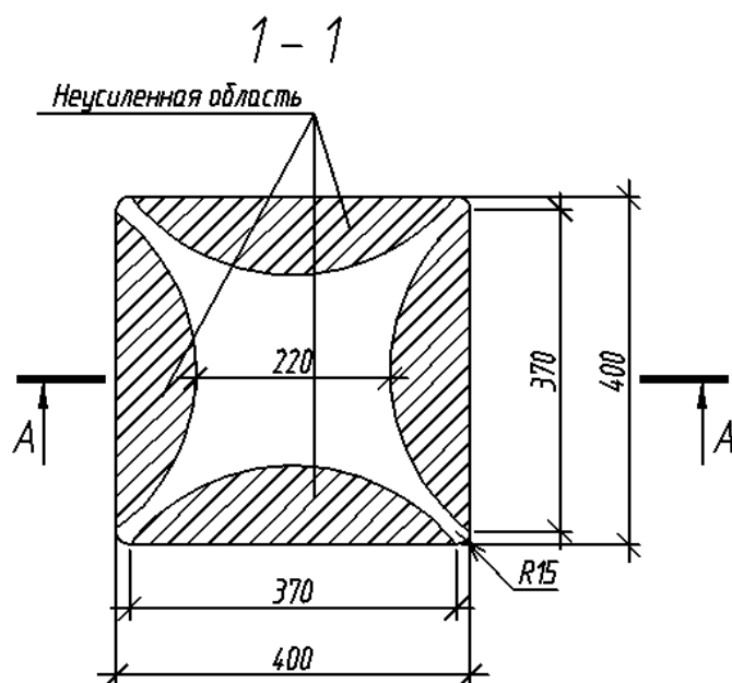
Рисунок В5 – Сечение колонны 1-1
