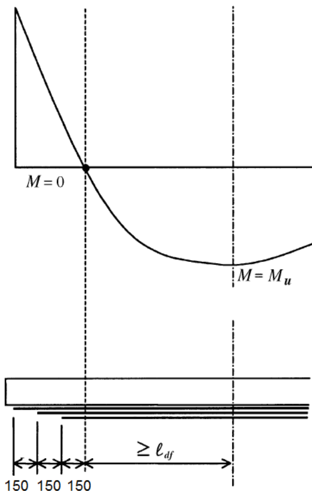
Рисунок 20 – Схема анкеровки многопролетных железобетонных конструкций
