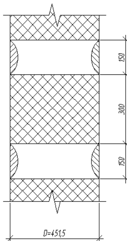
Рисунок В8 – Схема усиления круглой колонны
