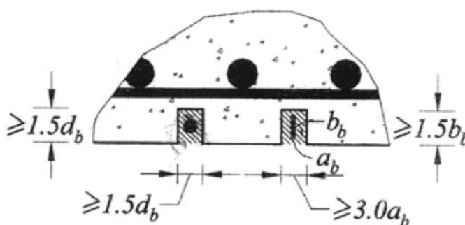
Рисунок 14 – Минимальные размеры пазов для установки композиционных материалов
