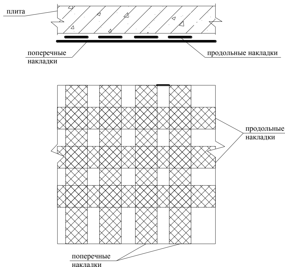
Рисунок 7 – Схема внешнего армирования плиты
