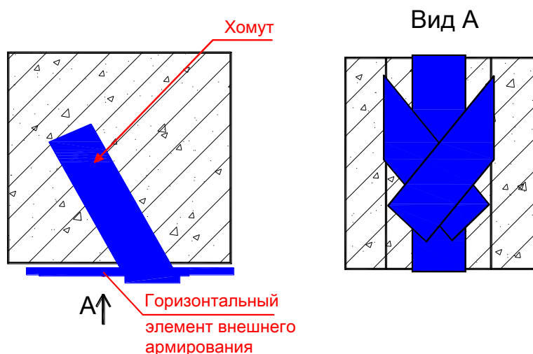
Рисунок 30 – Схема установки наклонных хомутов в балочных конструкциях
