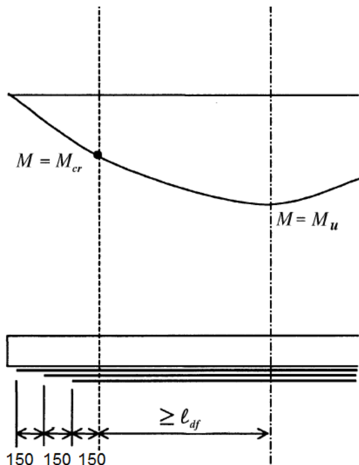
Рисунок 19 – Схема анкеровки однопролетных железобетонных конструкций
