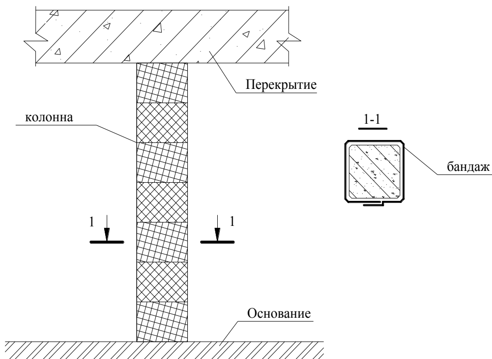
Рисунок 11 – Схема внешнего армирования колонны
