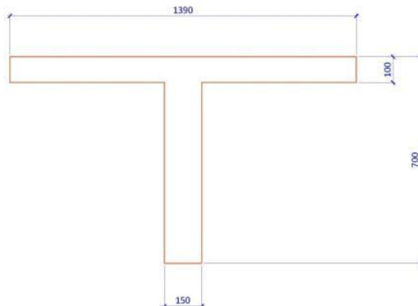
Рисунок Б.3 – Расчетное сечение балки
