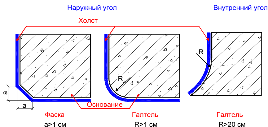
Рисунок 28 – Подготовка углов конструкции перед приклеиванием холстов
