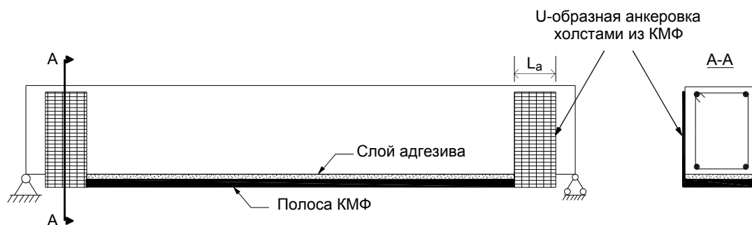
Рисунок 8 – Анкеровка концевых участков полосы композиционного материала
