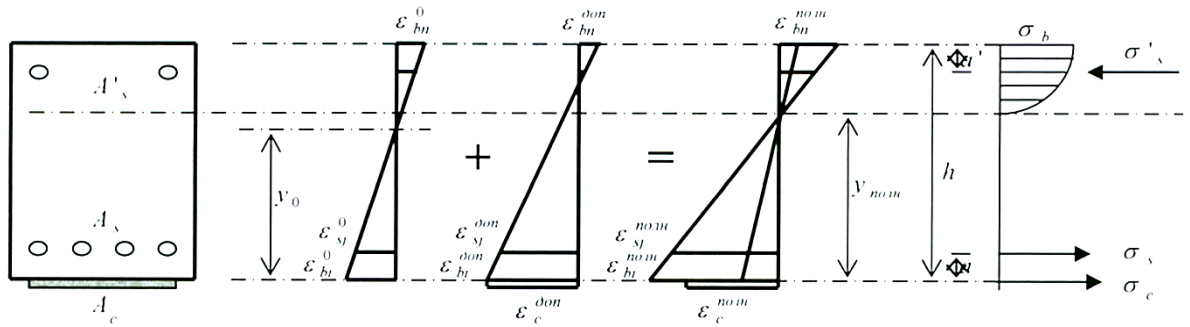
Рисунок 24 – Расчетная схема деформационной модели
