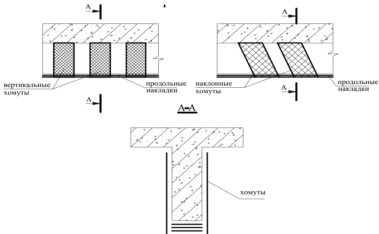
Рисунок 6 – Схема внешнего армирования балки
