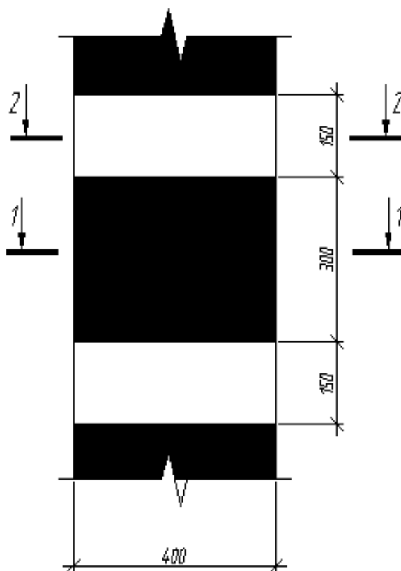
Рисунок В4 – Схема внешнего армирования квадратной колонны
