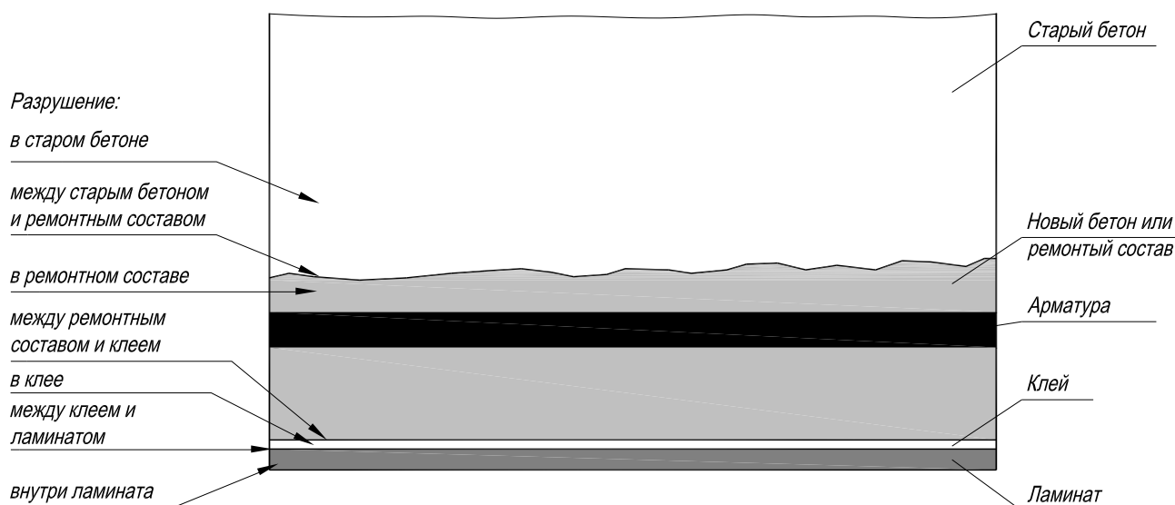
Рисунок 15 – Возможные поверхности разрушения усиливаемой (ремонтируемой) конструкции
