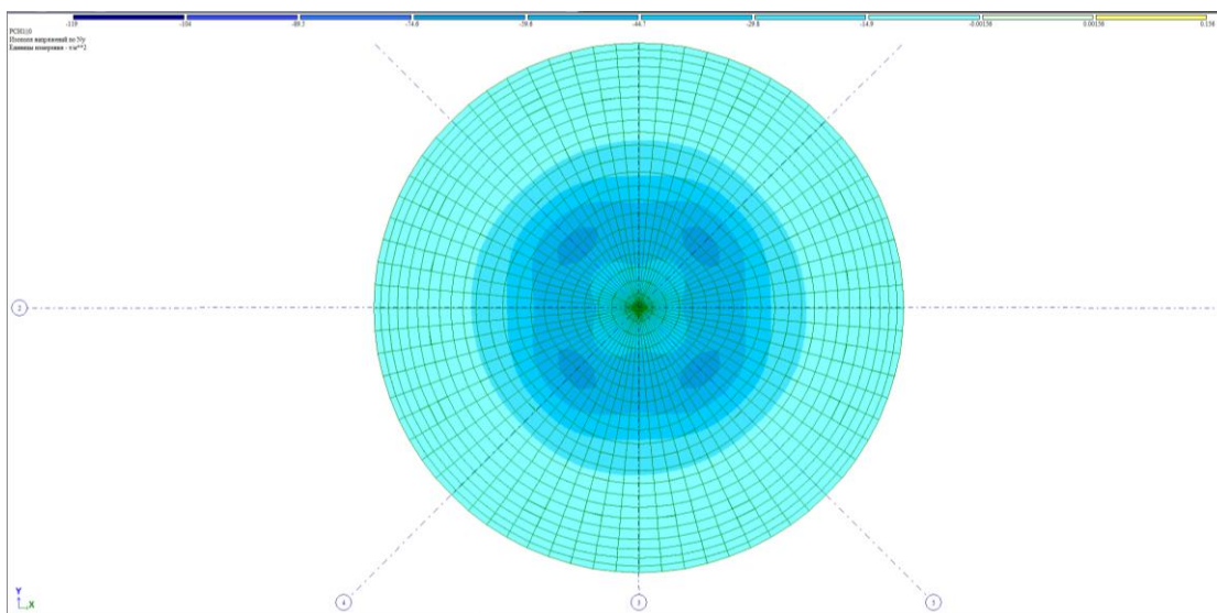
Рисунок Г5 – Мозаика напряжений N_y
