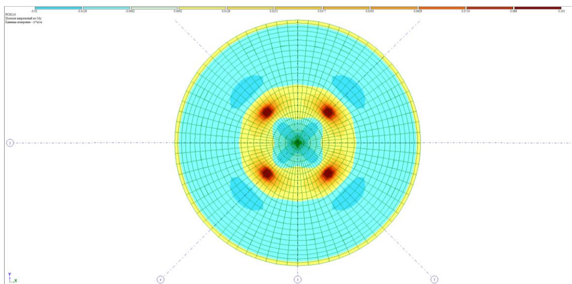
Рисунок Г3 – Мозаика напряжений M_y
