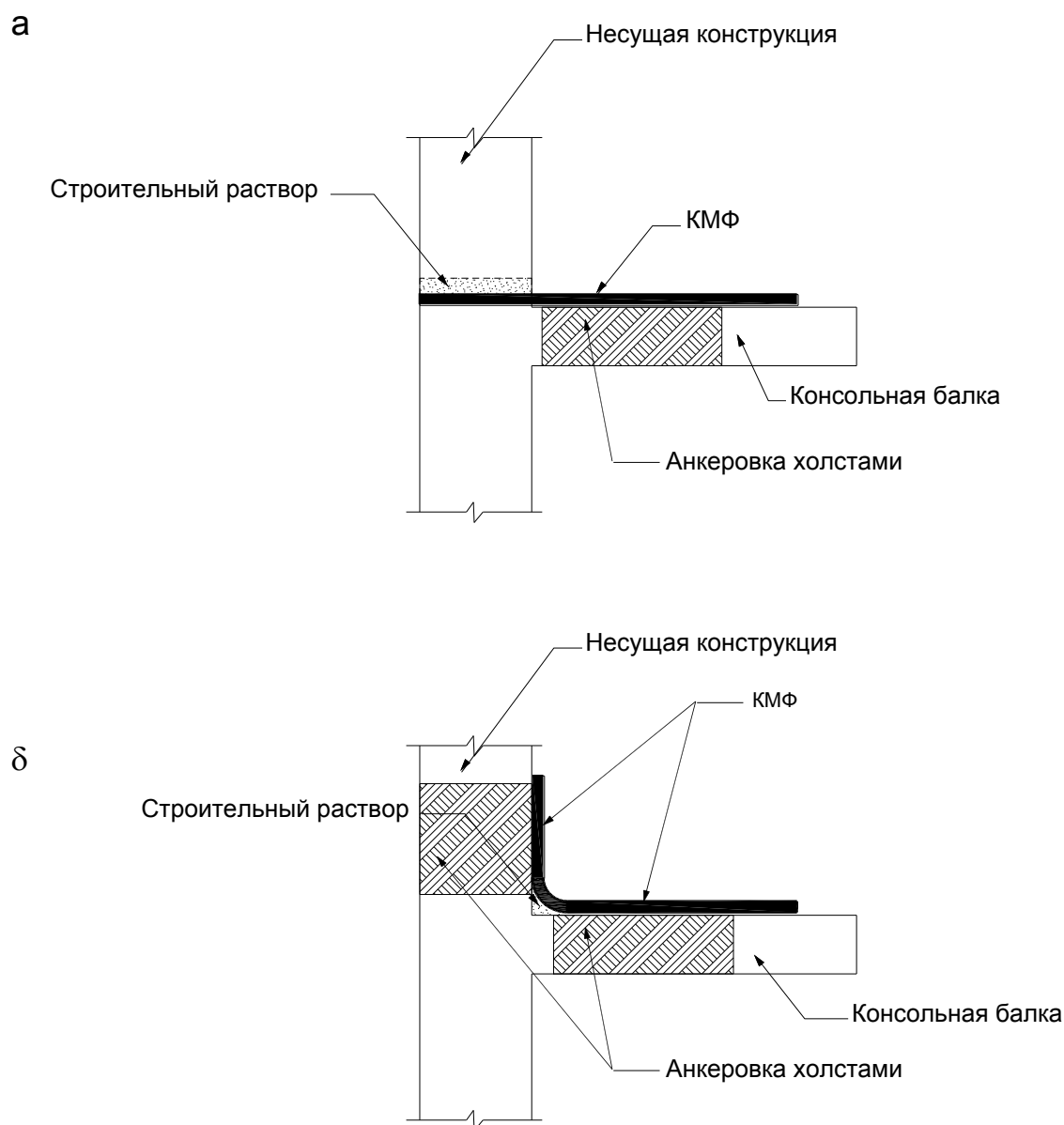
Рисунок 8 – Анкеровка концевых участков полосы композиционного материала
