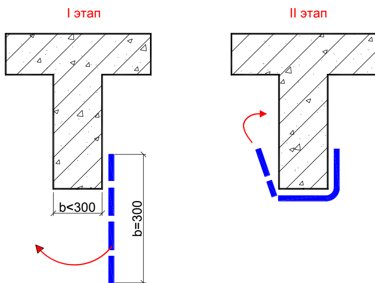
Рисунок 31 – Внешнее армирование балочных конструкций.
