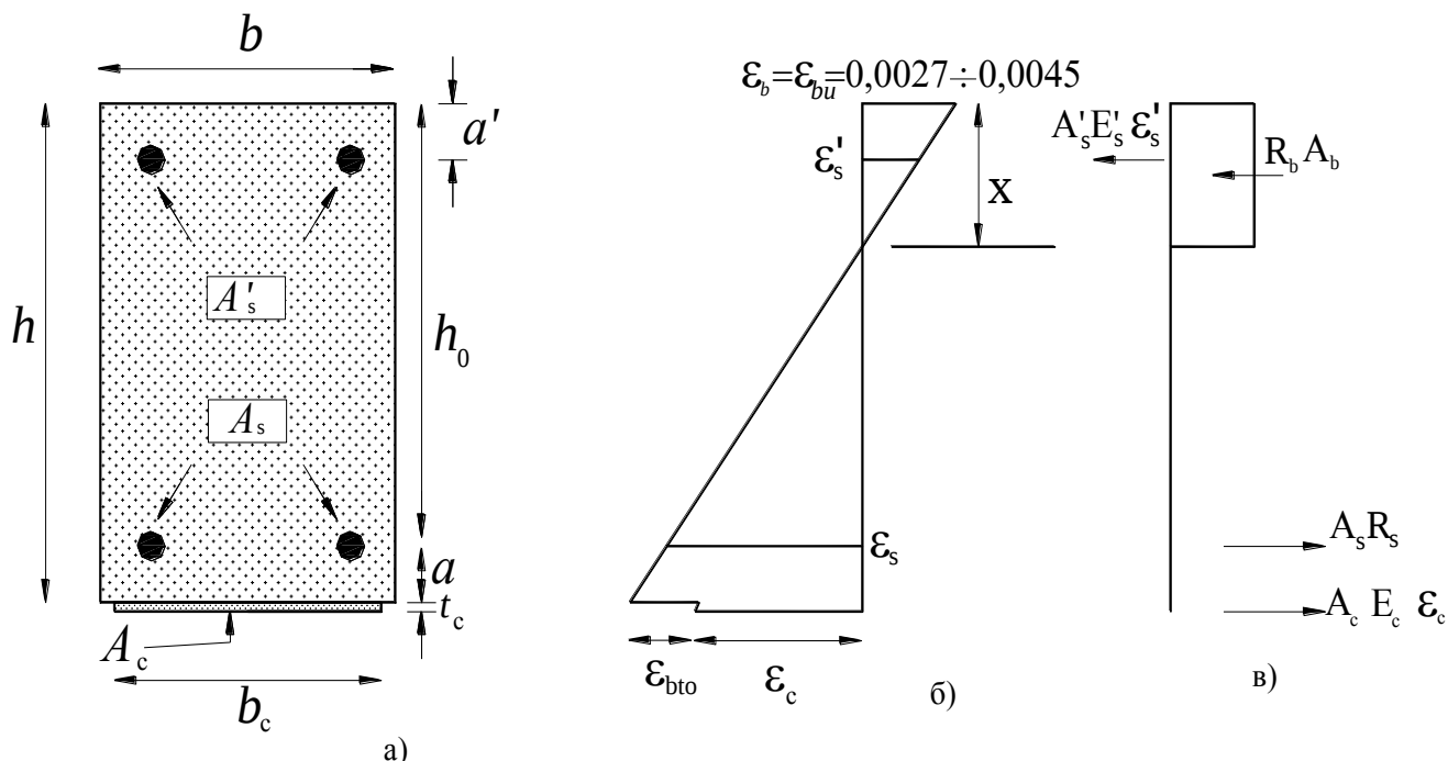
Рисунок 22 – Напряженно-деформированное состояние усиленного КМФ изгибаемого железобетонного элемента: a – поперечное сечение; б – распределение деформаций; в – распределение внутренних усилий
