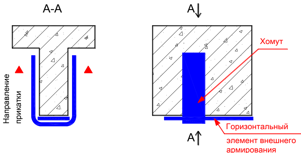
Рисунок 29 – Схема установки вертикальных хомутов в балочных конструкциях
