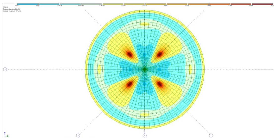
Рисунок Г2 – Мозаика напряжений M_x
