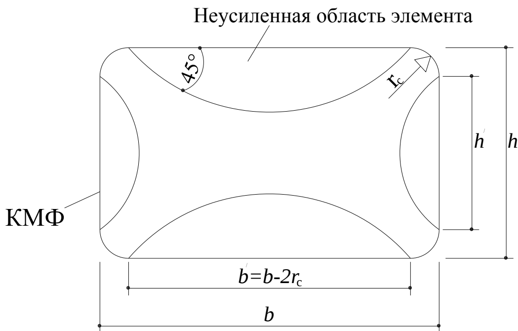
Рисунок 25 – Эффективная область усиления обоями из КМФ прямоугольных железобетонных колонн: b и h – размеры сторон прямоугольной колонны; b' и h' – размеры частей колонн, не охваченных усилением
