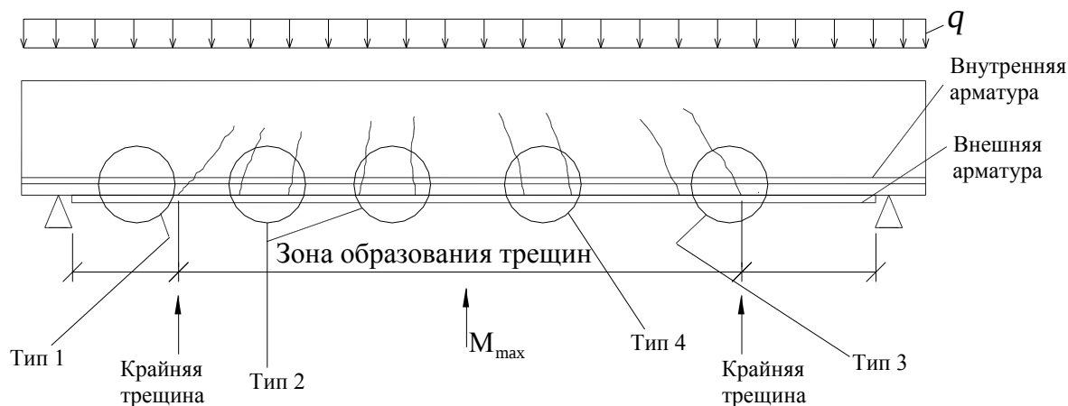
Рисунок 16 – Типы разрушения железобетонной конструкции, усиленной полосой композита
