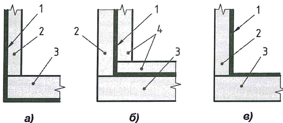
а) наружная гидроизоляция; б) гидроизоляция сэндвичного типа; в) внутренняя гидроизоляция 1 - гидроизоляционный материал; 2 - наружная стена сооружения; 3 - фундаментная плита; 4 - прижимные конструкции
