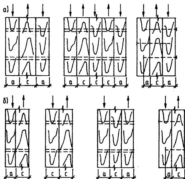
Рисунок 9 — Нагельные соединения
