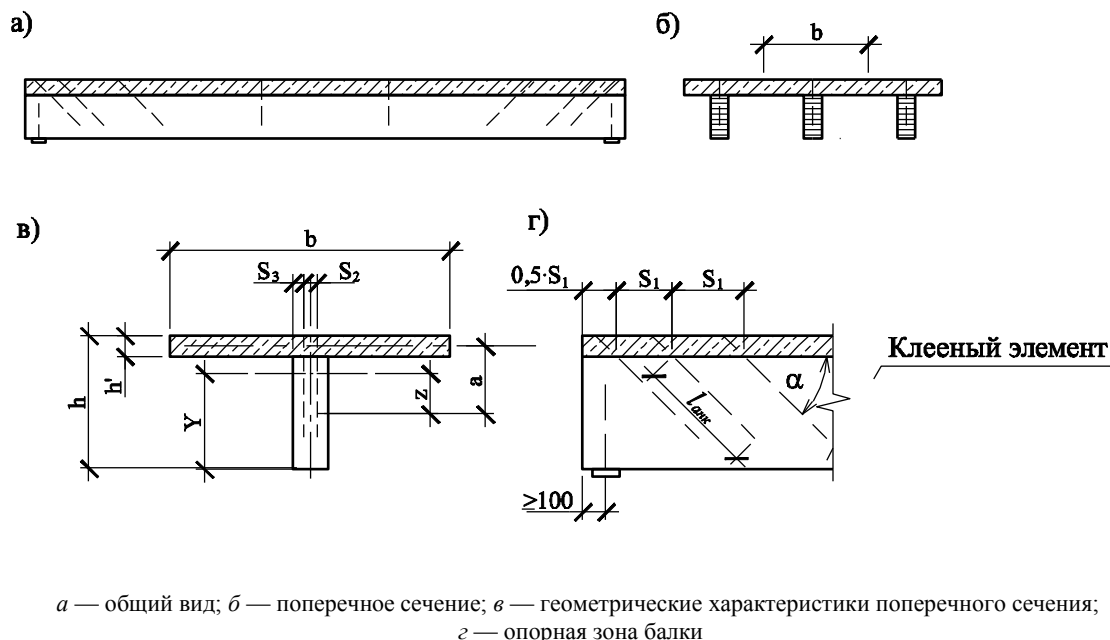
Рисунок 22 — Балка композитного сечения
