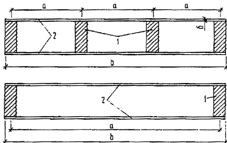
1 — продольные ребра; 2 — обшивка
