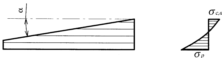
Рисунок 21 — Односкатная балка
