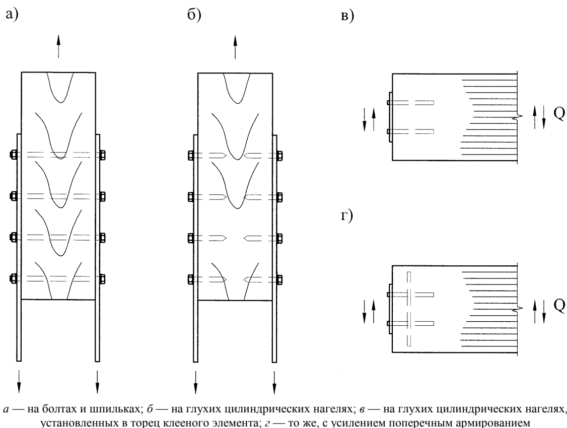
Рисунок 10 — Нагельные соединения со стальными накладками
