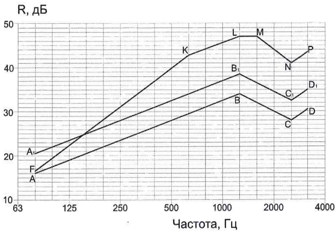
Рисунок А.2 - Расчетная частотная характеристика
