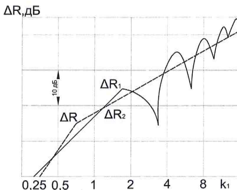
Рисунок В.1 - Дополнительная звукоизоляция двойным ограждением без жесткой связи по контуру
